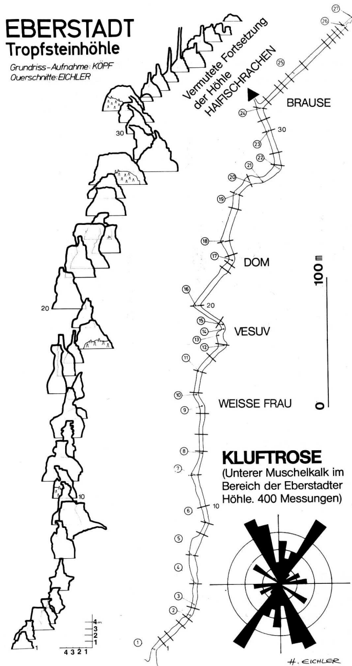
Abb. 1 Höhlenplan der Eberstadter Tropfsteinhöhle (Kreise geben Vermessungspunkte an).
